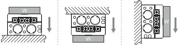
Fig. 1 : Applied load
