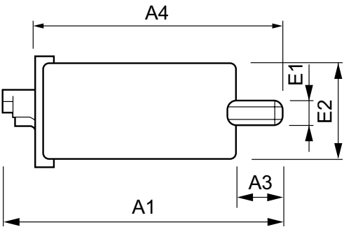
Bản vẽ kích thước
